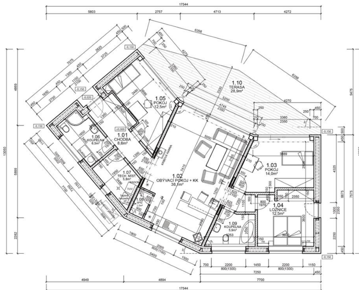
PUDORYS 1.NP
